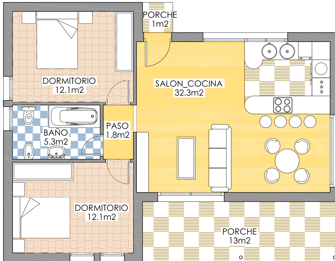
PLANTA BAJA
